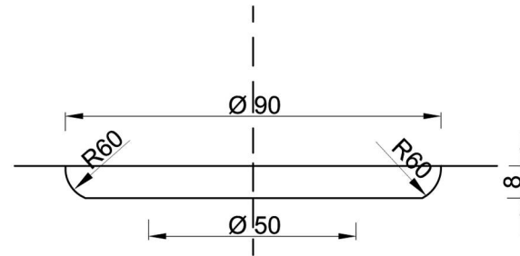
DETAIL A 10:1
